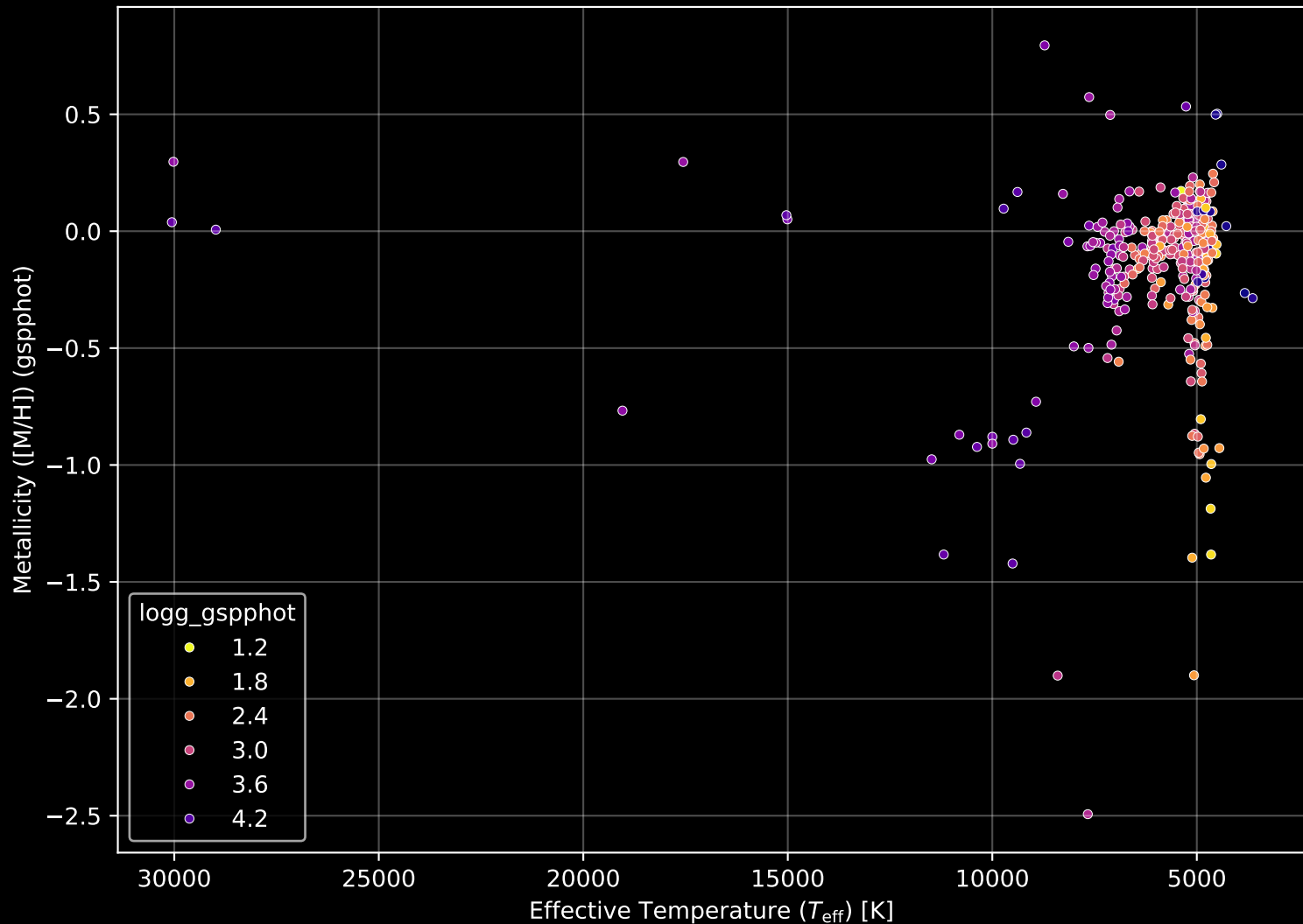
APOGEE DR17 Field: [188+00] Stellar Population Parameters (n= 348)
